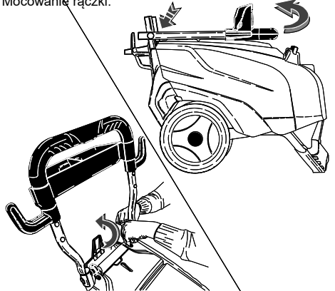
Mocowanie rączki.
